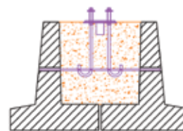
système de fondation articuler
